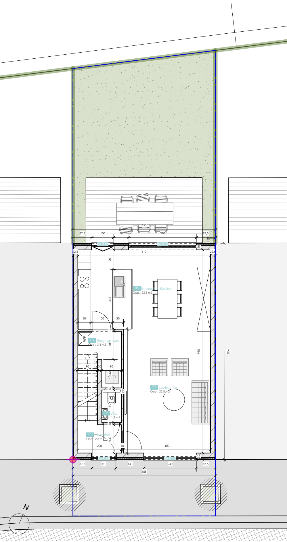
Gelijkvloers 65,20 m 2 | schaal 1:100
