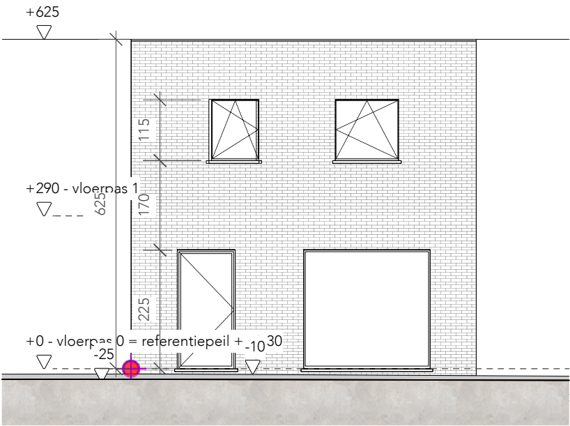
Zuidgevel | schaal 1:100
