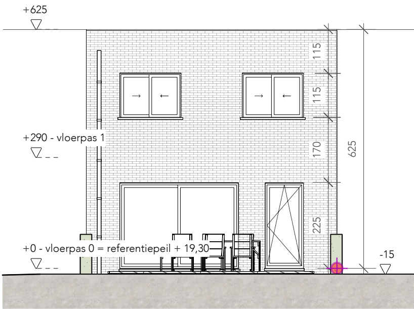
Noordgevel | schaal 1:100
