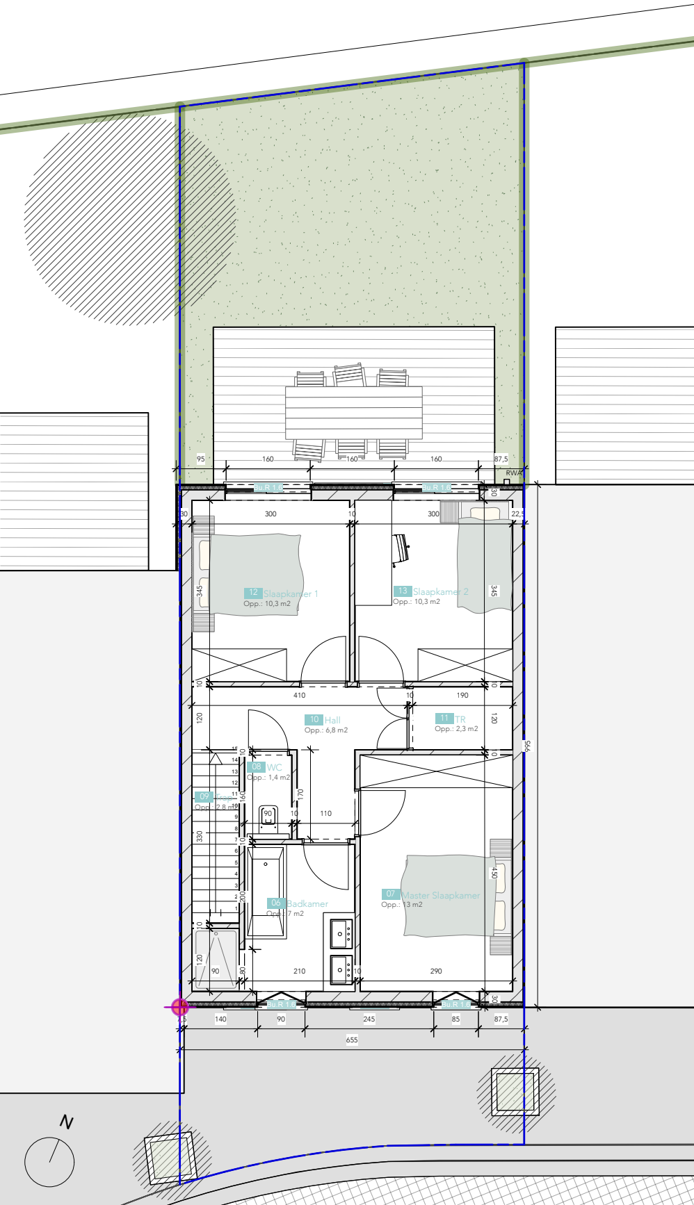
Verdieping 65,30 m² | schaal 1:100
