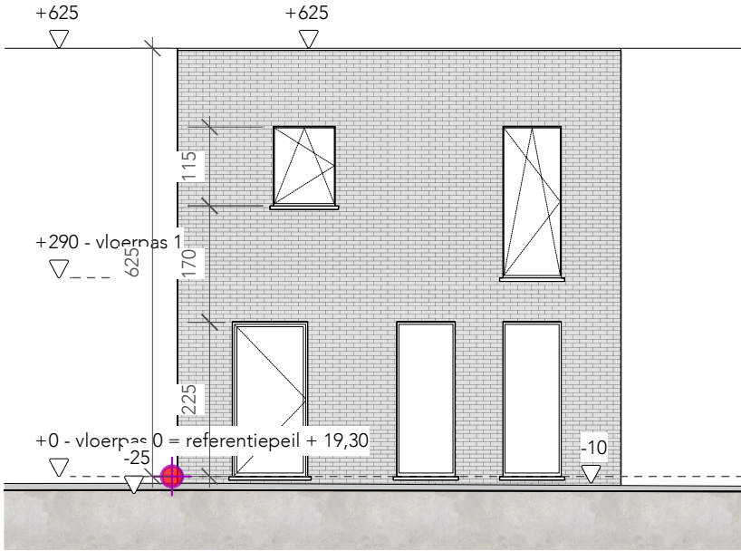
Zuidgevel | schaal 1:100
