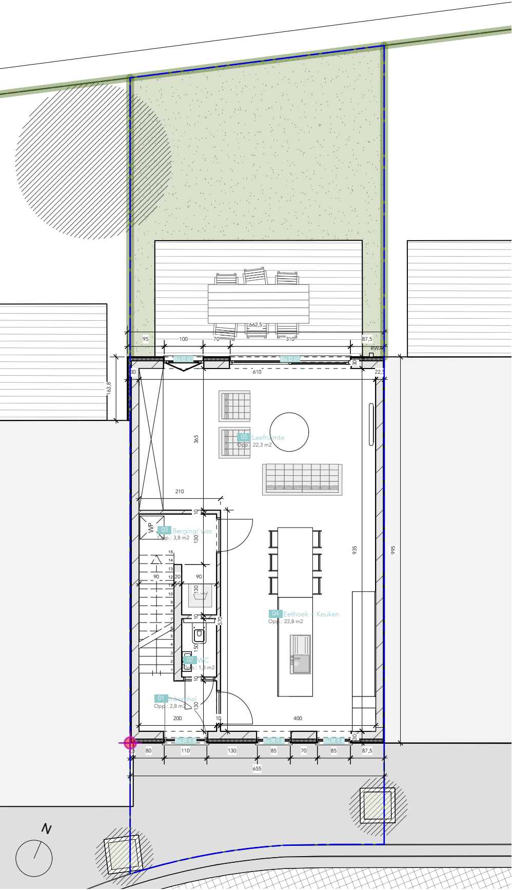
Gelijkvloers 65,30 m² | schaal 1:100
