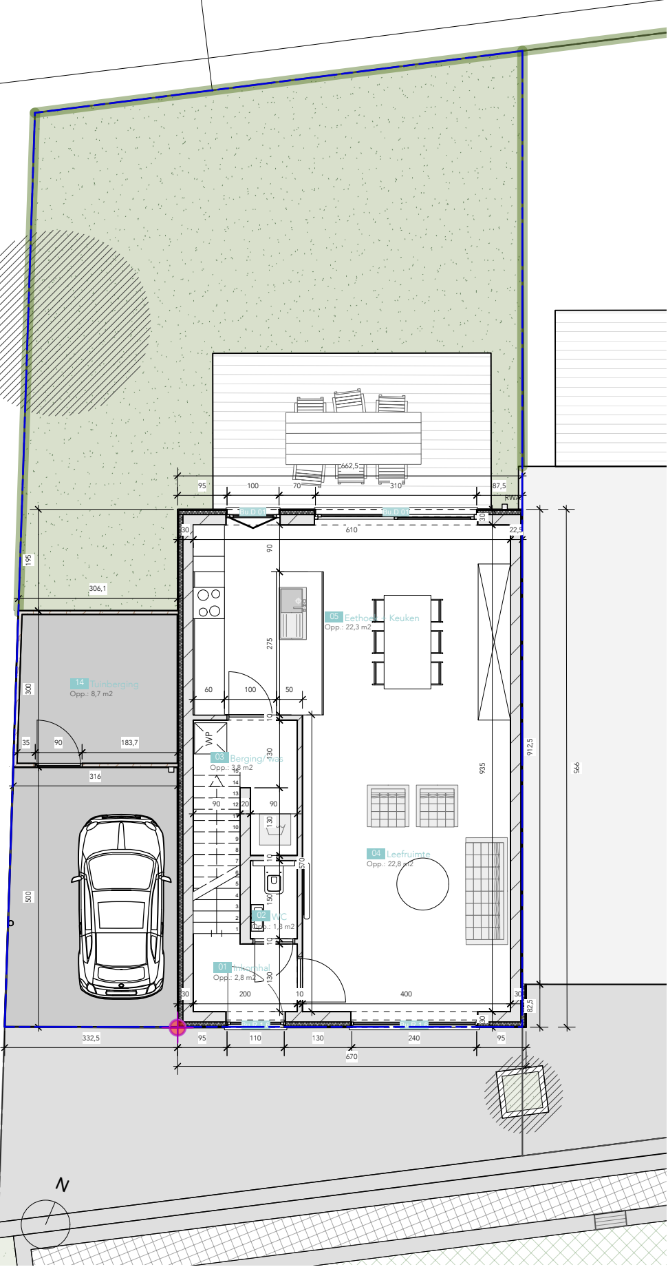
Gelijkvloers 75,30 m² | schaal 1:100
