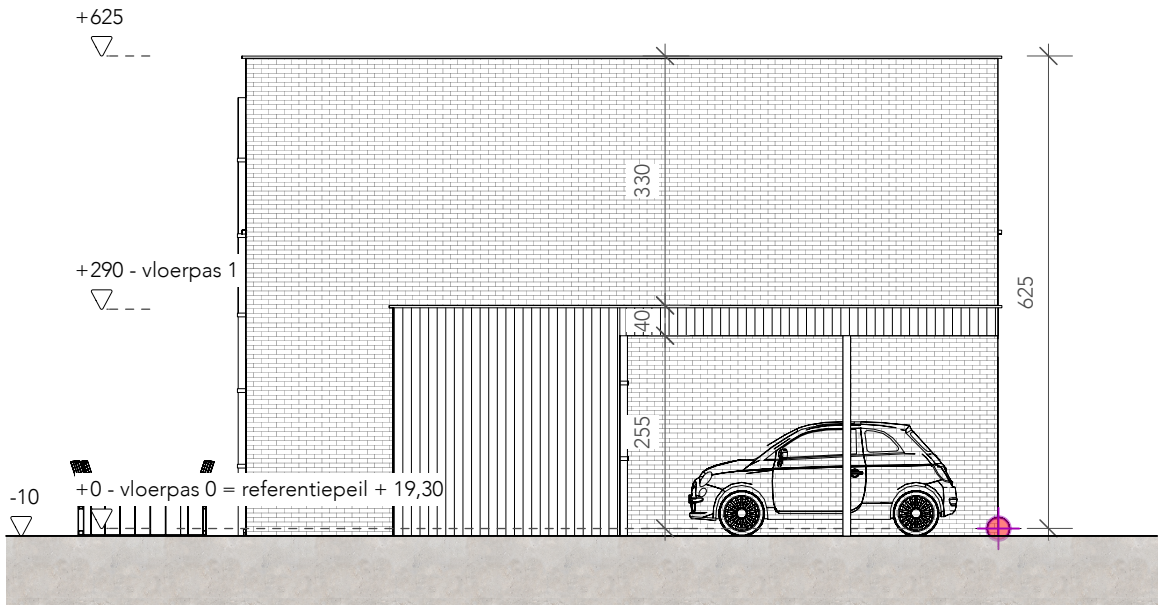
Westgevel | schaal 1:100
