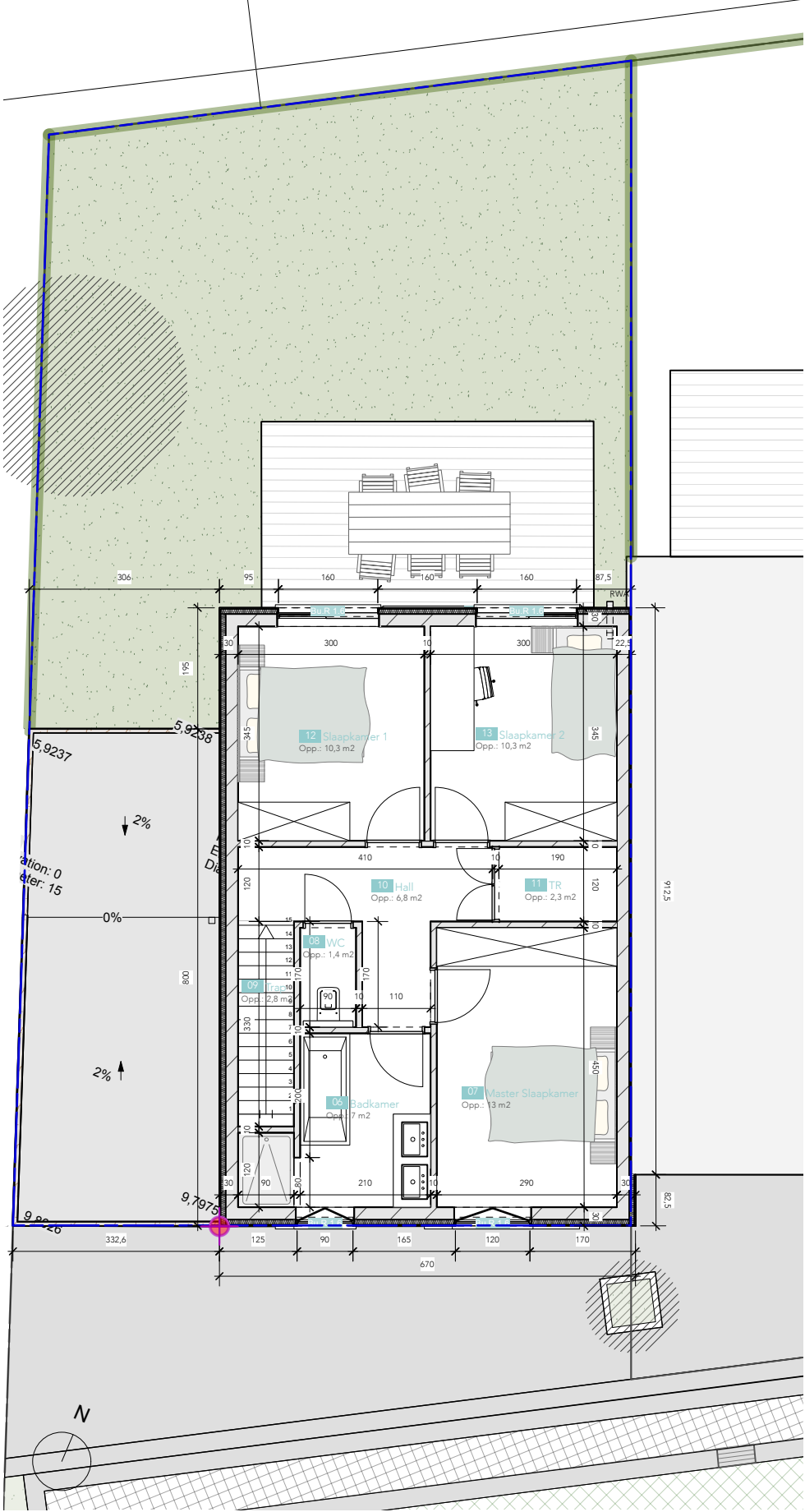
Verdieping 66,00 m² | schaal 1:100
