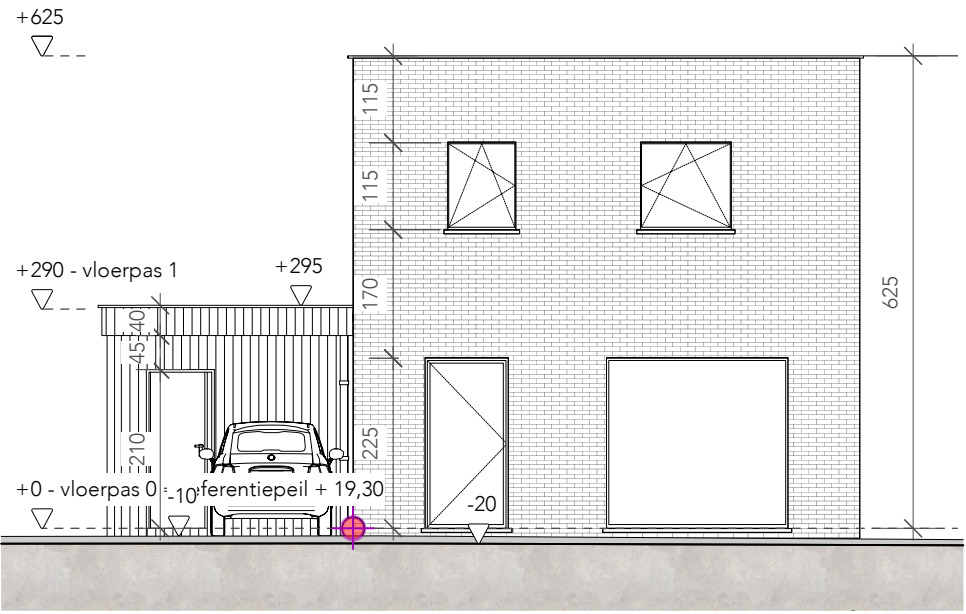
Zuidgevel | schaal 1:100
