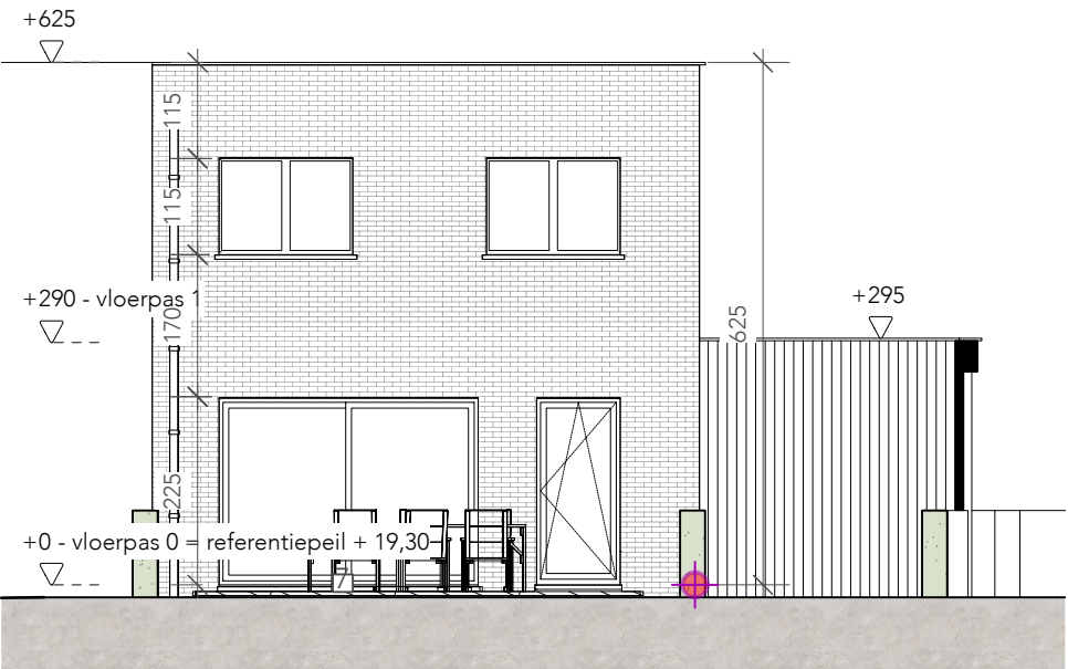
Noordgevel | schaal 1:100
