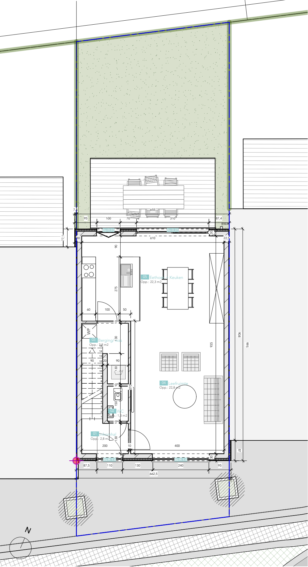
Gelijkvloers 65,30 m 2 | schaal 1:100
