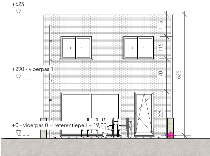
Noordgevel | schaal 1:100
