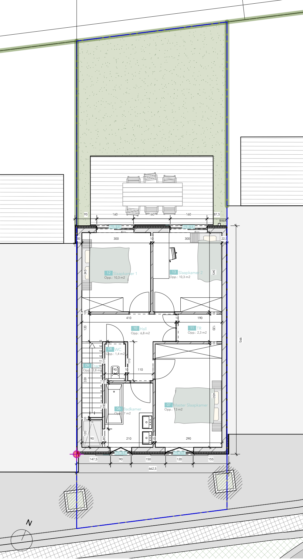
Verpieping 65,30 m 2 | schaal 1:100
