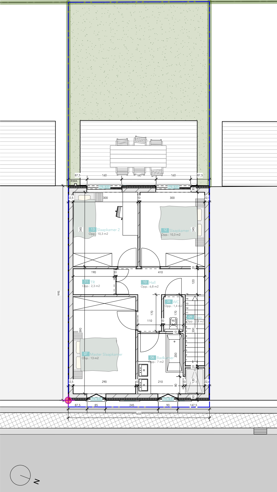
Verpieping 65,20 m 2 | schaal 1:100
