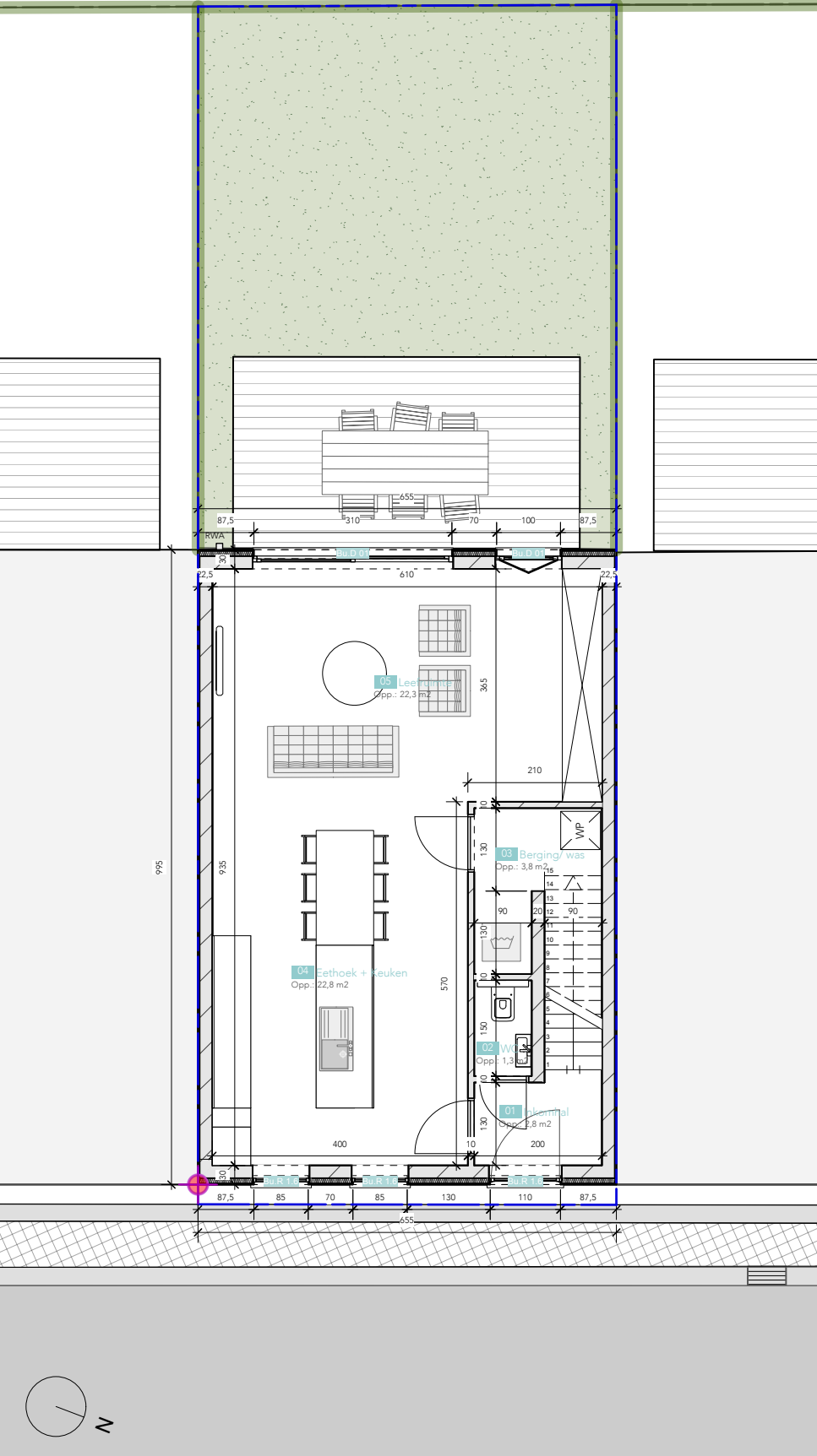
Gelijkvloers 65,20 m 2 | schaal 1:100
