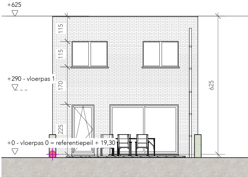
Westgevel | schaal 1:100
