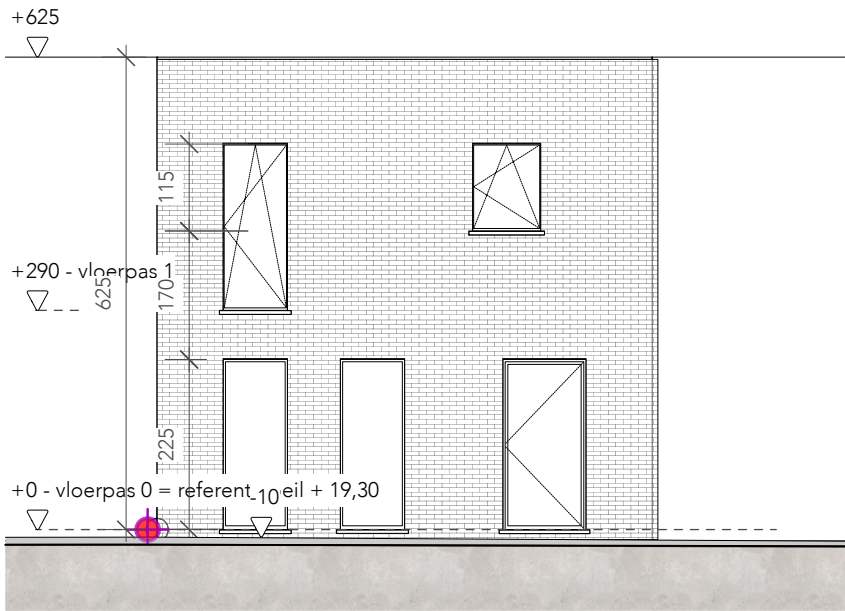
Oostgevel | schaal 1:100
