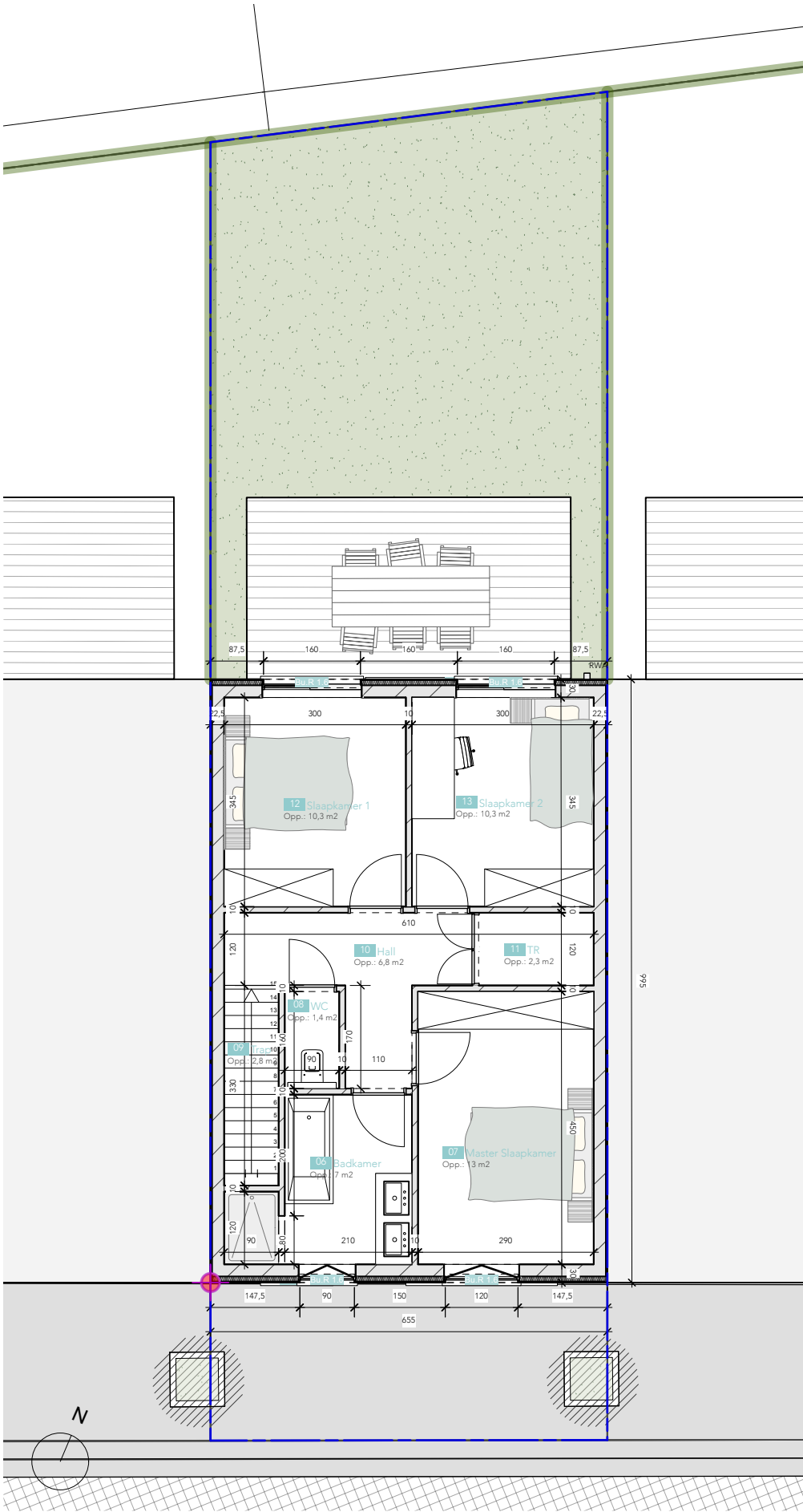
Verpieping 65,20 m² | schaal 1:100
