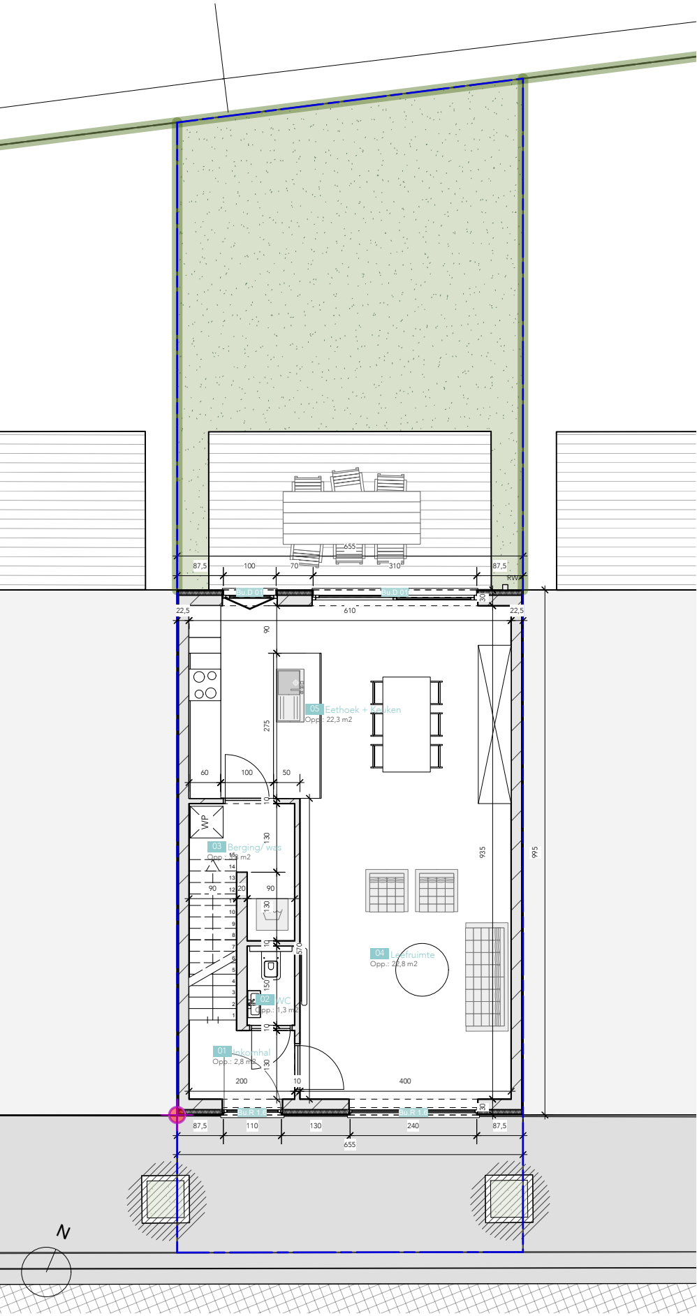
Gelijkvloers 65,20 m² | schaal 1:100
