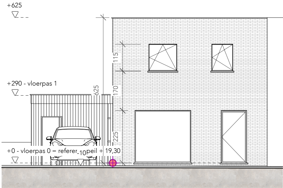
Oostgevel | schaal 1:100
