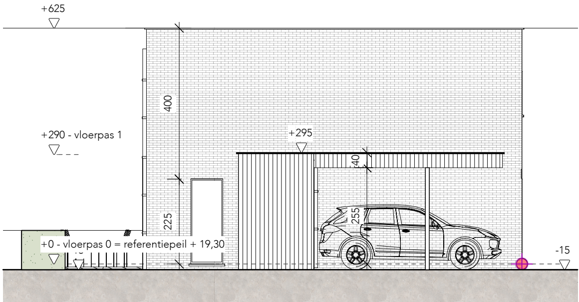
Zuidgevel | schaal 1:100
