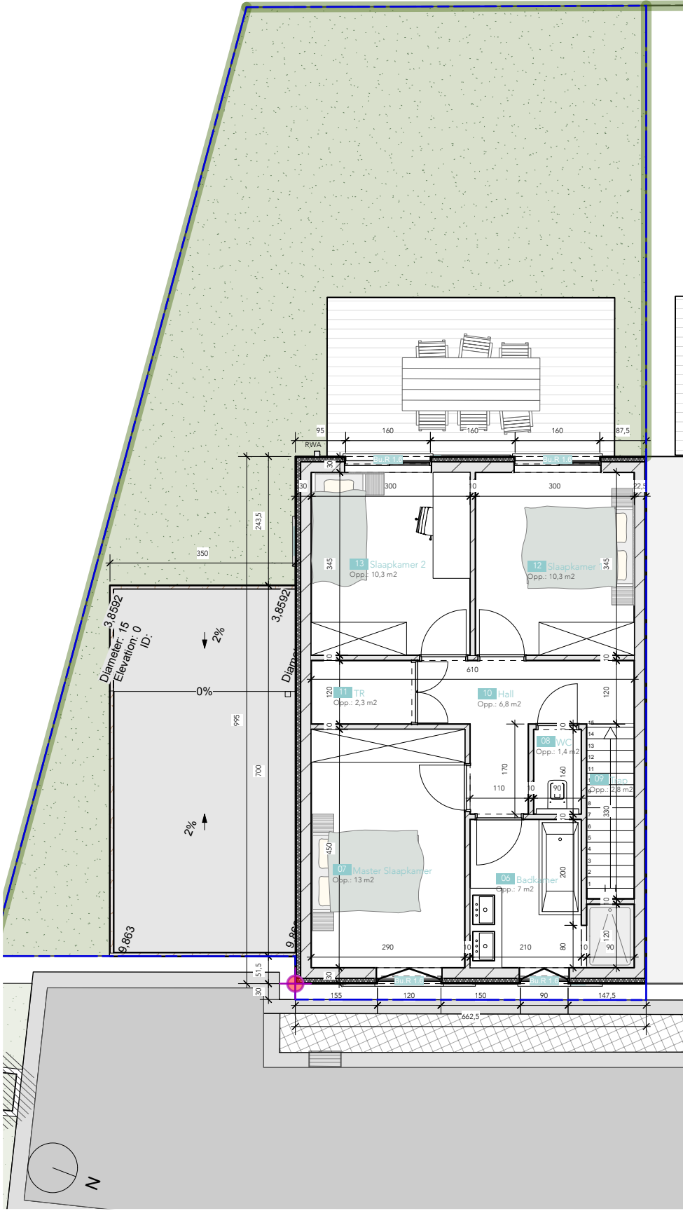
Verdieping 65,90 m² | schaal 1:100
