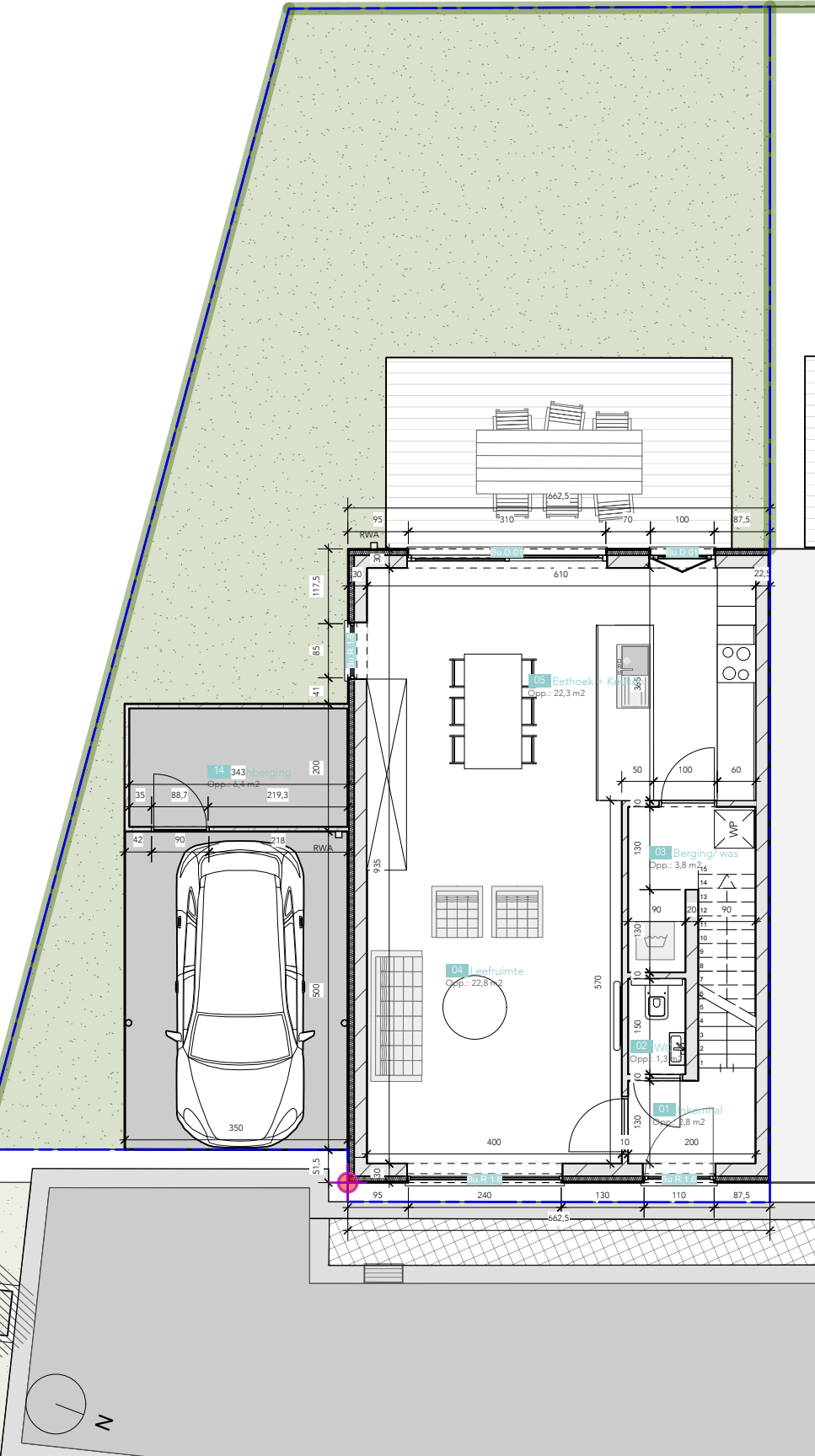
Gelijkvloers 72,90 m² | schaal 1:100
