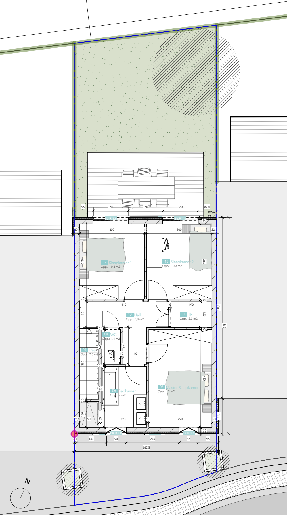
Verpieping 65,40 m² | schaal 1:100
