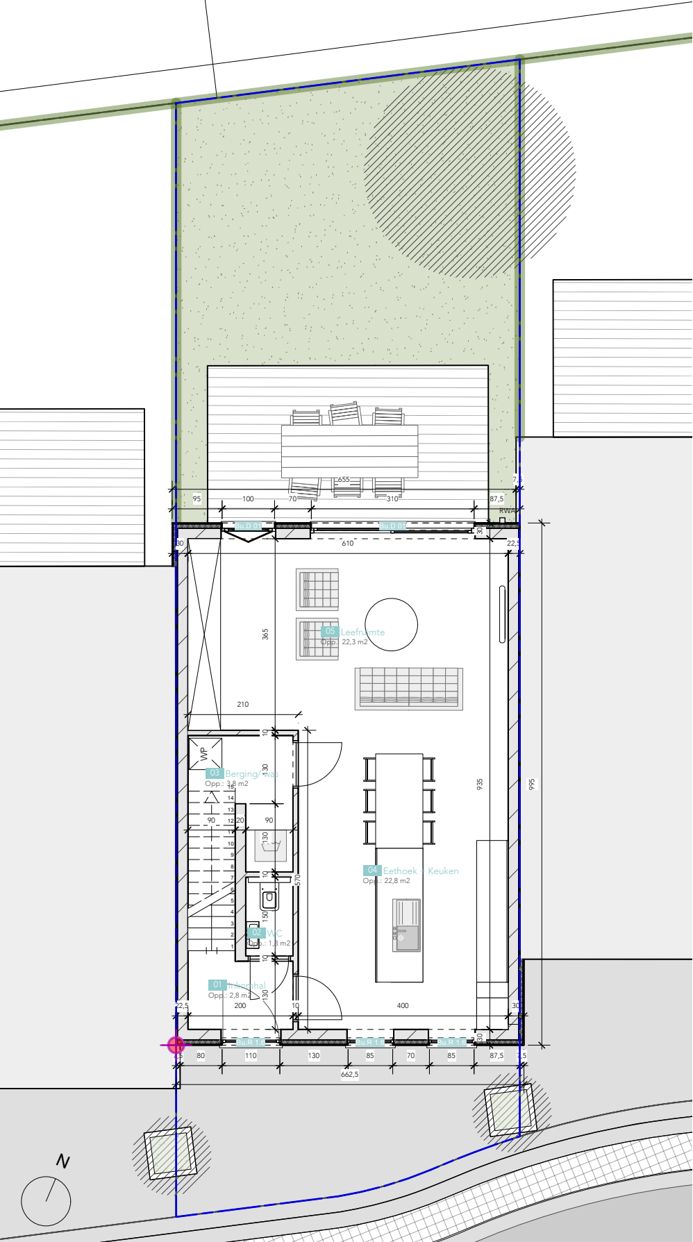
Gelijkvloers 65,40 m² | schaal 1:100
